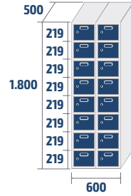
ECOZ-30/2 PRO COD: 47115 48,4kg · 0,54m 3
