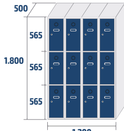
ECOM-30/4 PRO COD: 47049 66,8kg · 1,08m 3
