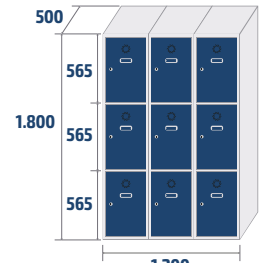
ECOM-40/3 PRO COD: 47053 60,6kg · 1,08m 3
