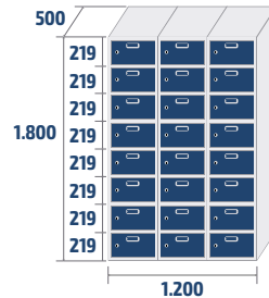
ECOZ-40/3 PRO COD: 47121 82,7kg · 1,08m 3
