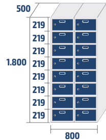
ECOZ-40/2 PRO COD: 47120 56,8kg · 0,72m 3
