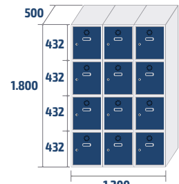
ECOC-40/3 PRO COD: 47070 65,1kg · 1,08m 3
