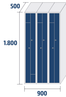
ECOL-30/3 PRO COD: 35303 61,3kg · 0,81m 3
