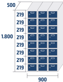
ECOZ-30/3 PRO COD: 47116 70,1kg · 0,81m 3
