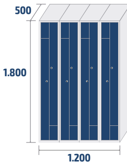
ECOL-30/4 PRO COD: 35304 79,8kg · 1,08m 3
