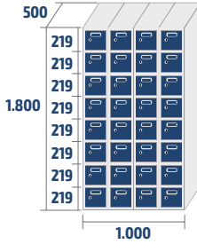
ECOZ-25/4 PRO COD: 47112 82,6kg · 0,9m 3
