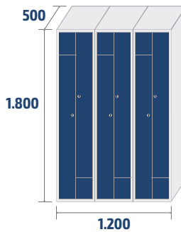
ECOL-40/3 PRO COD: 35403 72,3kg · 1,08m 3
