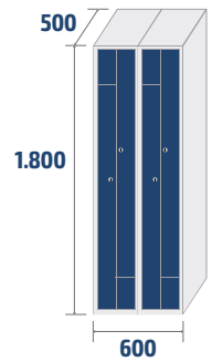
ECOL-30/2 PRO COD: 35302 42,9kg · 0,54m 3
