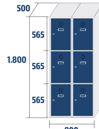
ECOM-40/2 PRO COD: 47052 42,4kg · 0,72m 3
